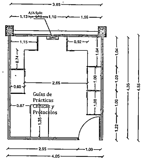
PLANTA DIMENSIONADA PROPUESTA 1
